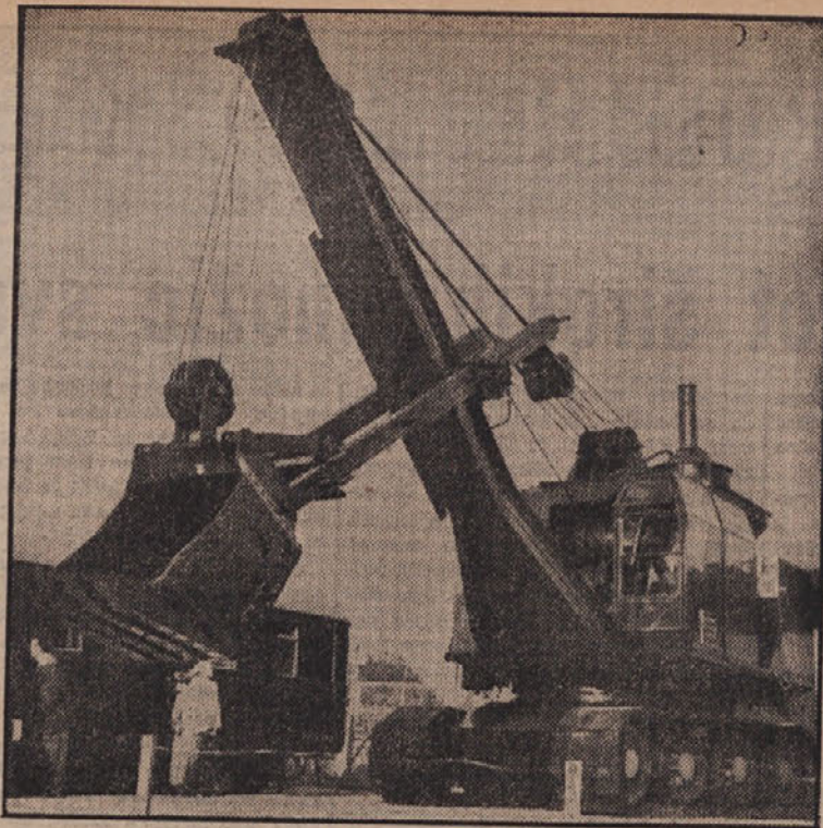
Mogočen parni bager jugoslovanske konstrukcije in proizvodnje
