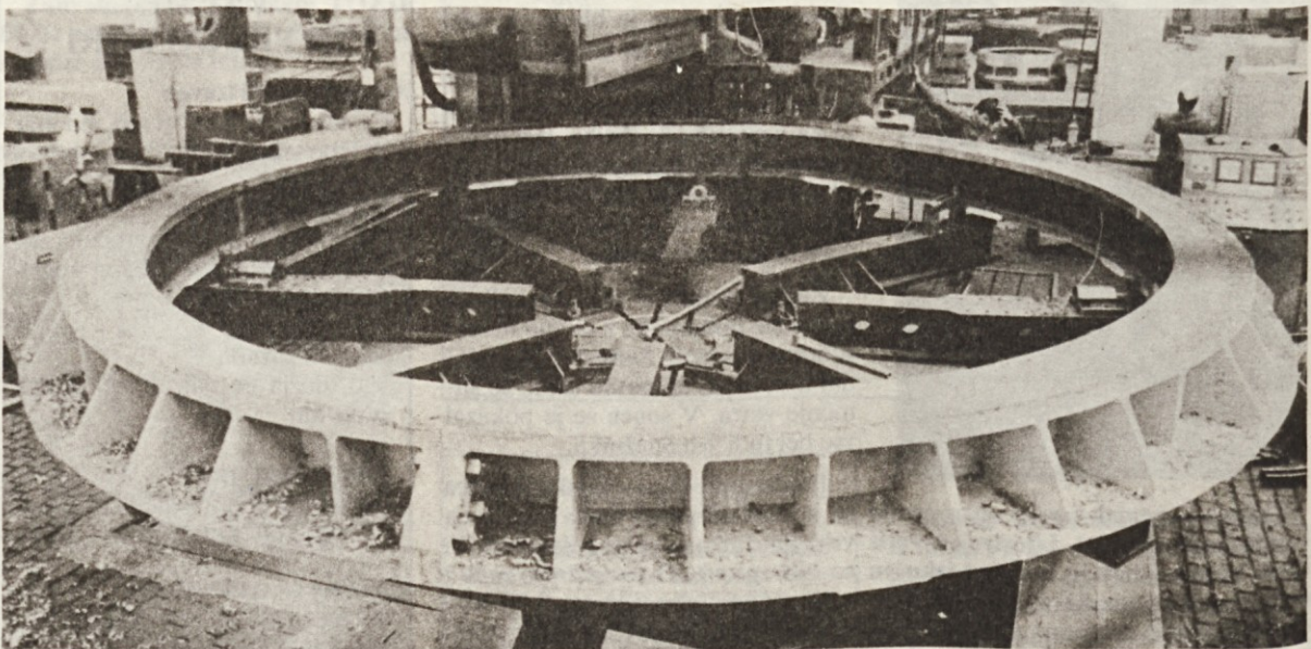
Spodnji vodilnikov obroč za HE Mavčiče. Premer obroča je 7060/ mm in visok 440 mm. (Foto: K. G.)
