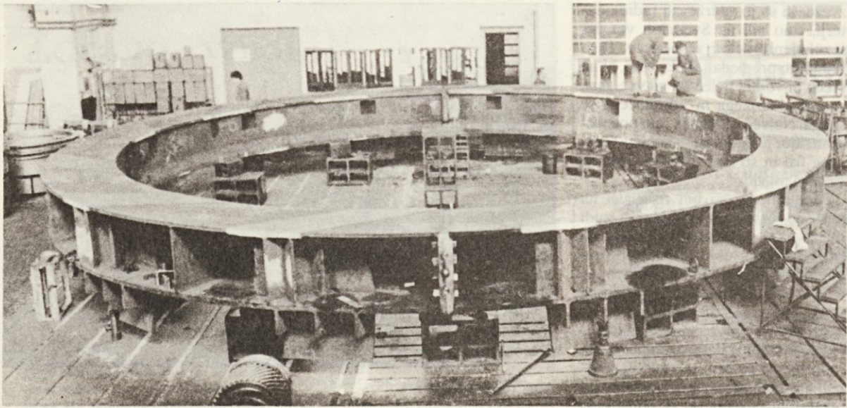
Predvodilni obroč za HF Haditha v pripravi za nadaljnjo montažo. Zunanji premer obroča je 12 metrov, njegova celotna teža pa bo 96 ton (Foto: K. G.)
