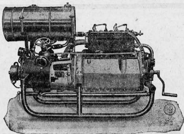
Dvocilindrska motorna brizgalnica, model 1929, 18/20 P. S., pritisk do 16 atm. Hladilnik novega sistema, ogrevanje črpalke s toplo čisto vodo.
