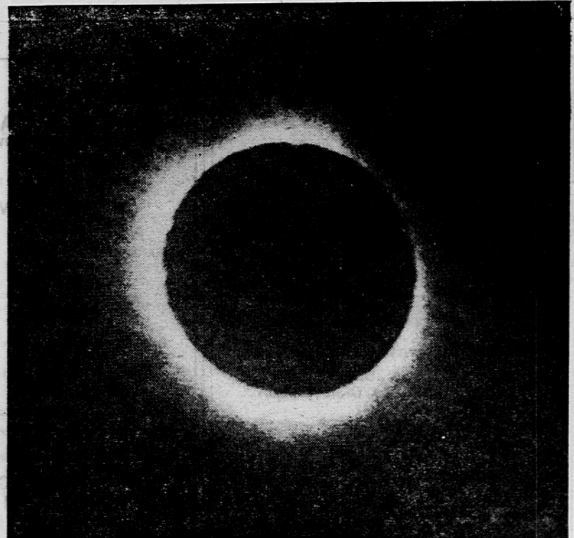
SONČNI MRK NAD JUŽNO AMERIKO — Z instrumenti v raketah in z drugimi modernimi pripomočki so astronomi mnogih dežel spremljali sobotni popolni sončni mrk, ki je bil viden v 82 km širokem pasu posevno čez srednji del južnoameriške celine. Podoben sončnega mrka na sliki so posneli v bližini Lime (Peru). Telefoto: UPI
