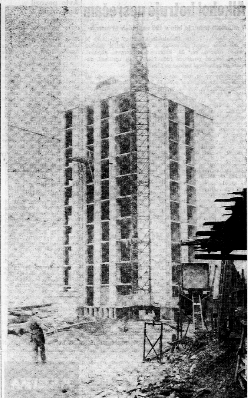
TRI STOLPNICE — 120 STANOVANJ — Gradbišče treh stolpičev in kotlarni na Viču v Bobenčevi ulici. Takih gradbišč s po nekaj deset ali največ dvesto, tristo stanovanj je razsutih širom po Ljubljani blizu petdeset. — Na tem gradbišču so tla močvirna in samo za pilotiranje enega stolpca je šlo 30 milijonov starih dinarjev. Razen tega je tod visoka potresna stopnja in za protipotresno gradnjo so morali uporabiti občutno več armiranega betona, kakor če bi te stolpce gradili denimo na Savskem polju. Za isti obseg investicij bi na prodnatem terenu ob Savi lahko zgradili kar kakih 10 stanovanj in v razen tega bi bila ta stanovanja lahko tudi cenejša. — Če bi na Ljubljano gledali kot na enoten gospodarski prostor, bi lahko na prodnatem Savskem polju v Šiški, za Bežigradom, v Mostah načrtovali in gradili naselja s tudi po več sto in tisoč stanovanj, kar bi omogočalo industrijsko gradnjo, proizvodnjo velikih serij raznih gradbenih elementov ipd. Foto: S. Busić
