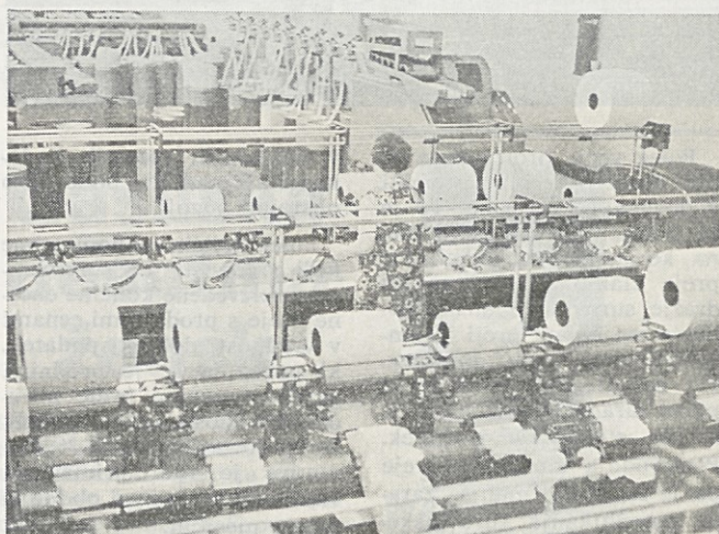
Proizvodnja česane preje bo trenutno upadla, ker bodo stroje prestavili v prizidek (slika levo), na njihovo staro mesto v predpredilnici (desna slika) pa bo prišel flyer krušik
