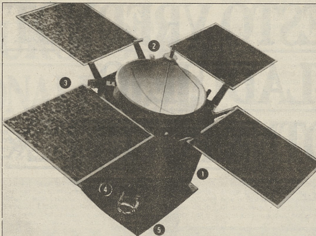
Vesoljska sonda NEAR: 1. ohišje sonde, 2. razprta antena (prečnik 1,5 m), 3. solarni paneli, 4. motor, 5. različni instrumenti
