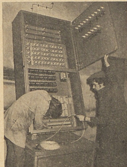
Montaža razdelilne omarice, izdelane za žičnico na Kaninu.
