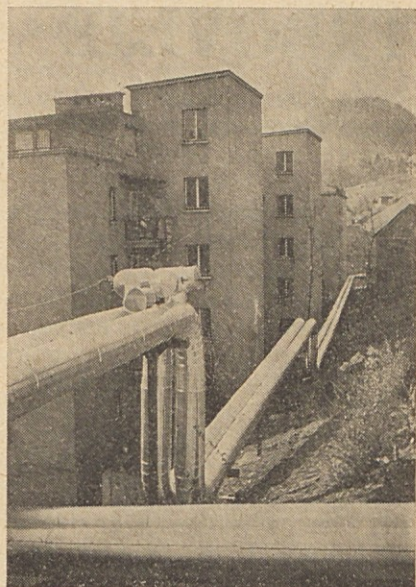
Odsek magistralnega toplovoda, ki poteka zadaj stanovanjskih blokov Cementarne Trbovlje ob Rudarski cesti. (Foto M. C.)
