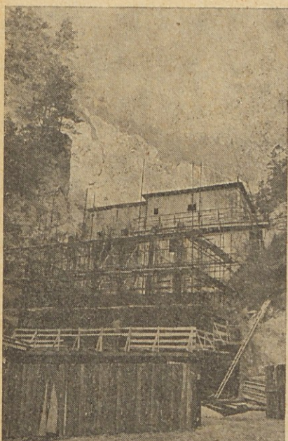
Kamnomol TOZD Rudnik premoga Hrastnik, v Hrastniku, v teku rekonstrukcijskih del.
