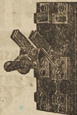
Ročni menjalnik s zavarovanjem, na dva pola. 250 Volt, do 400 Amperov.
