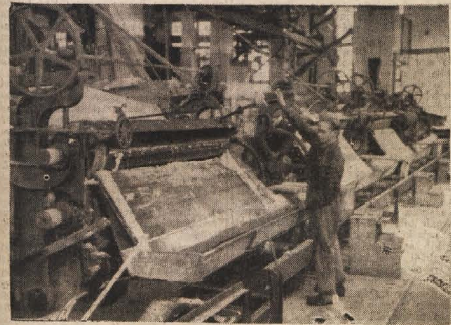
Stroji v brusilnem oddelku, kjer se dela lesovina, osnovna surovina za izdelavo papirja.
