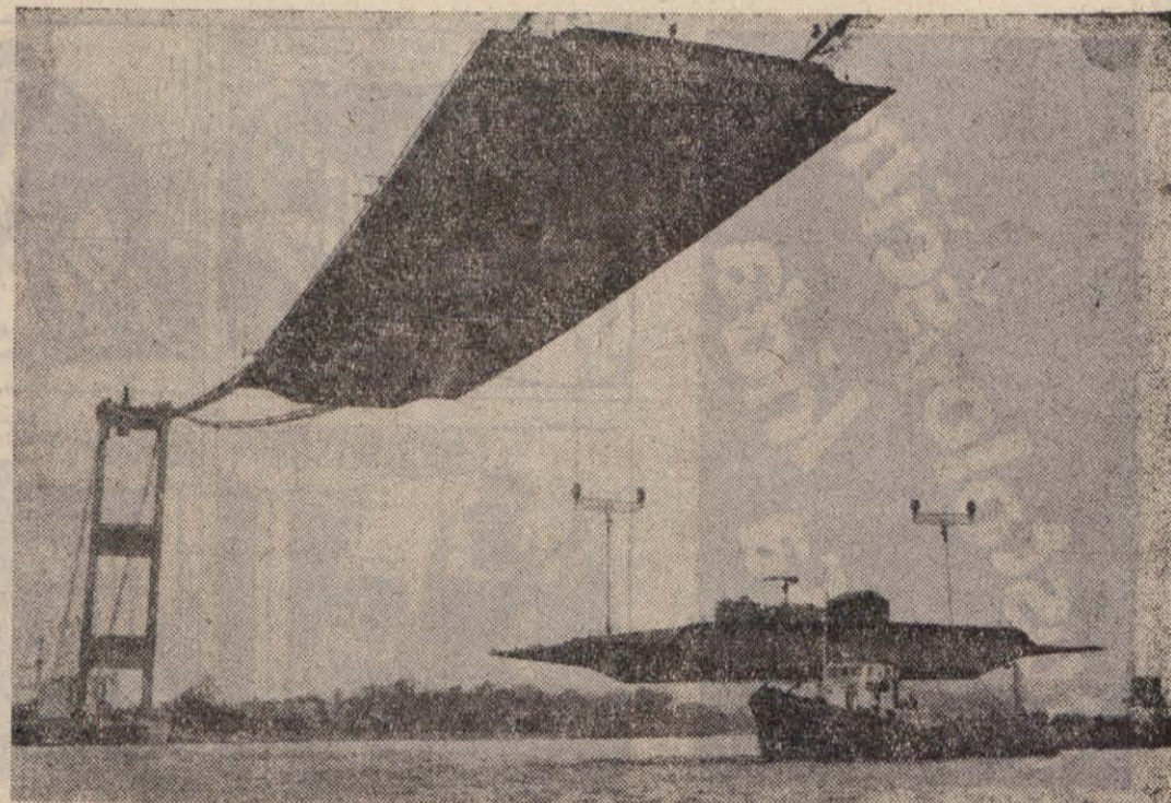
MOČNI škripci dvigujejo 190 ton težak del novega mostu na reki Severn v Angliji. Gre za novo tehniko pri gradnji mostov: jeklene dele mosta sestavijo na bregu in jih potem kar obesijo na nosilne kable.
