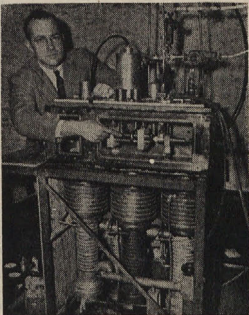
Pred kratkim smo poročali o atomski uri, ki so jo skonstruirali v Ameriki. Tu vidimo na sliki ta izum profesorja fizike Charlesa Townesa. (AND)
