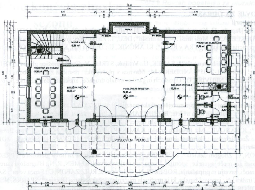
TLORIS PRITLIČJA
