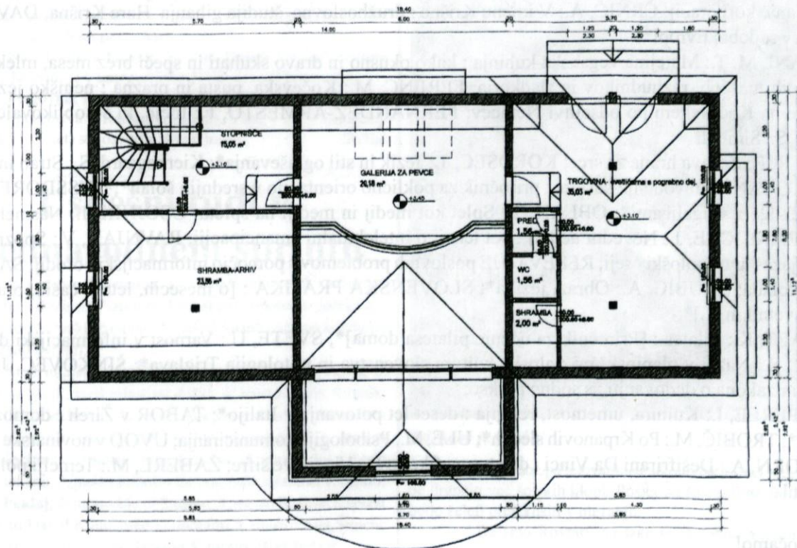
TLORIS MANSARDE
