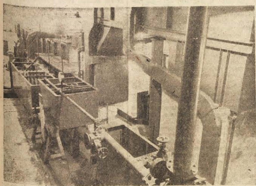
Pogled v laboratorij: na levi in na sredi model hidrocentrale na Zeti; na desni del »male« poskusne postaje
