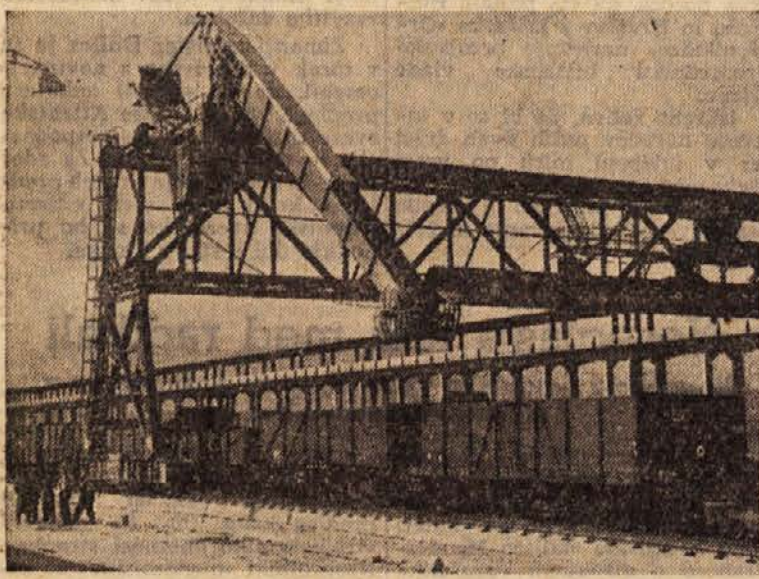
Vzdolž deponije premoga ob novi termoelektrarni Šoštanj se pomika velik portalni žerjav, ki opravlja vse manipulacije s premogom, bodisi da razmešča pripravljeni premog po deponiji ali pa ga z deponije dviga in prenaša do transportne naprave (na sliki v ozadju), odkoder ga s transportnimi trakovi spravijo do silosov na vrhu pogonske stavbe.
