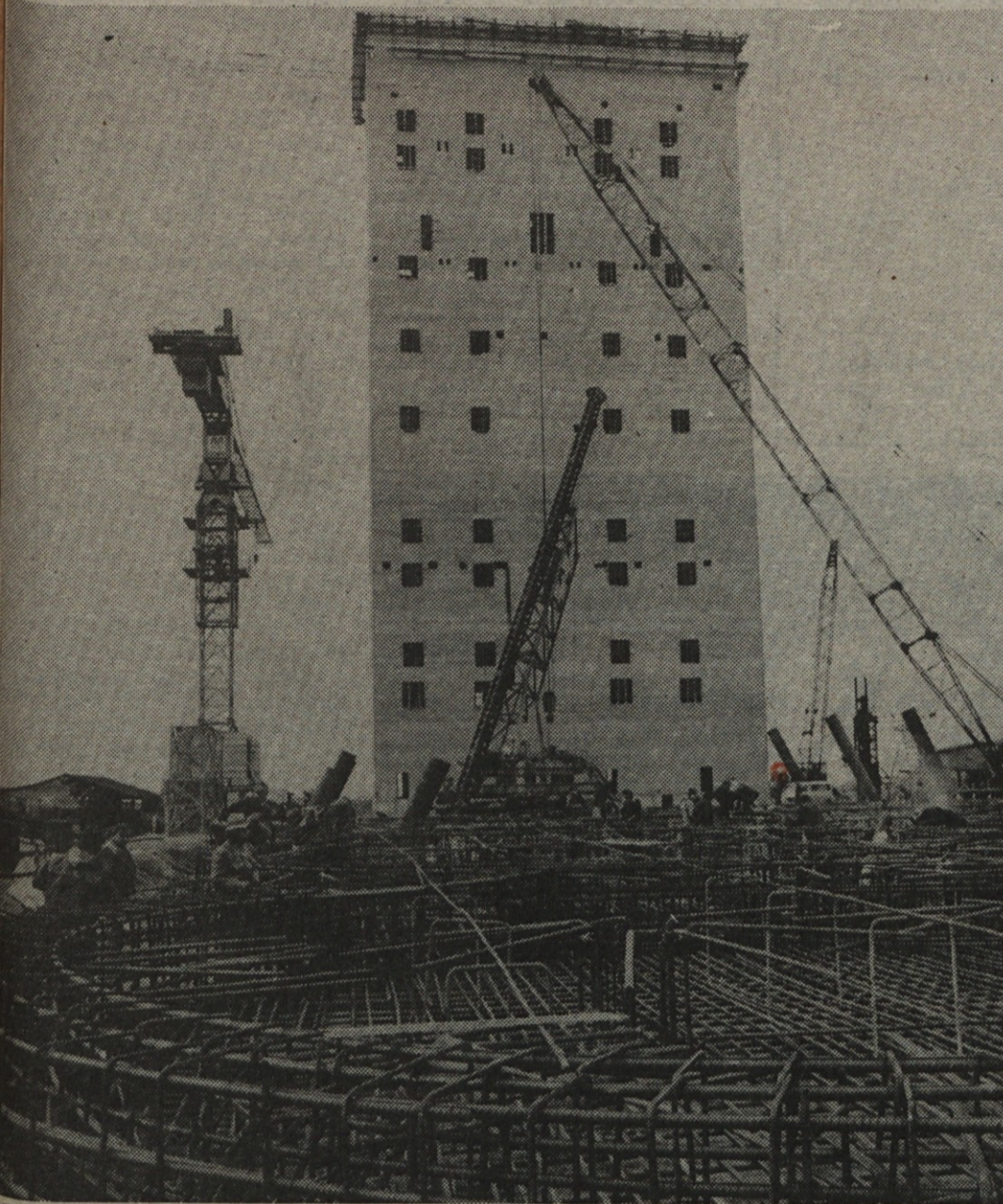
Gradnja 60.000 tonskega silosa v Luki Koper je bila zaupana Gradisu
