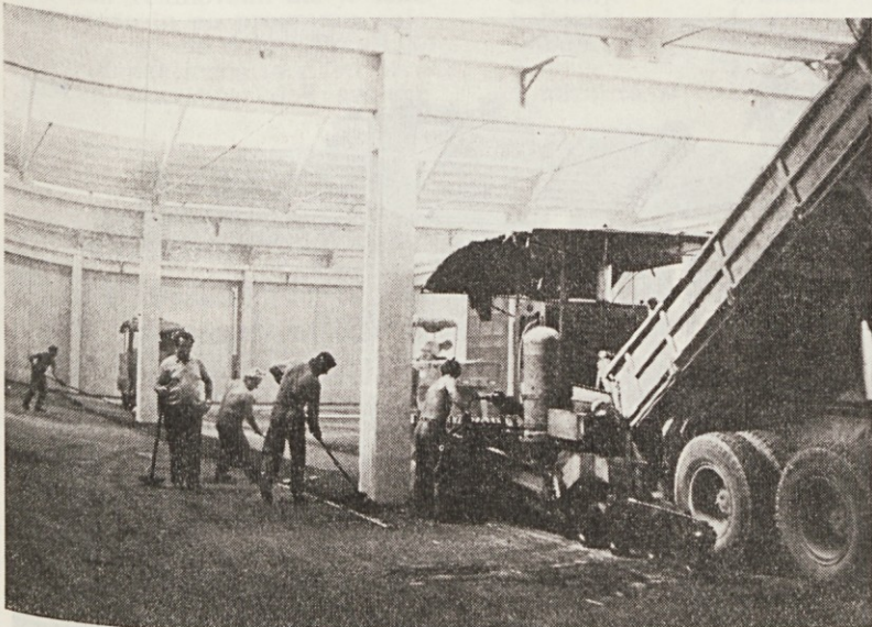
Asfaltiranje v novem skladišču gotovih izdelkov
