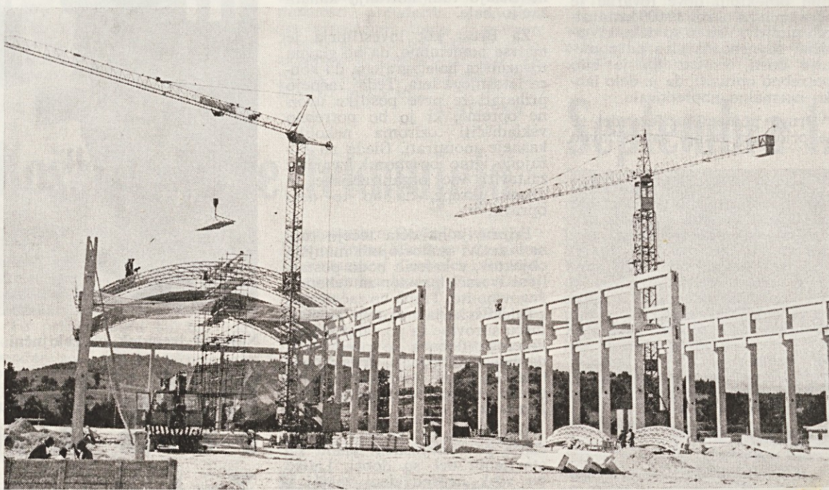
Nove naložbe — nove možnosti za gospodarski napredek
