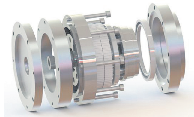
Planetni zobniški prenosnik, razvit v podjetju Podkrižnik (Foto: arhiv podjetja)
