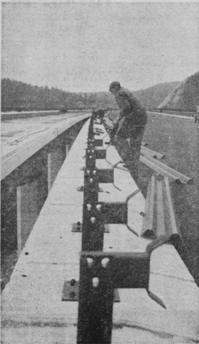
Montana iz Zaleca se je še posebej izkazala pri vertikalnem opremljanju cest. Posnetek je nastal pri montaži ograj na avtocesti Vrhnika—Postojna—Razdrto.
