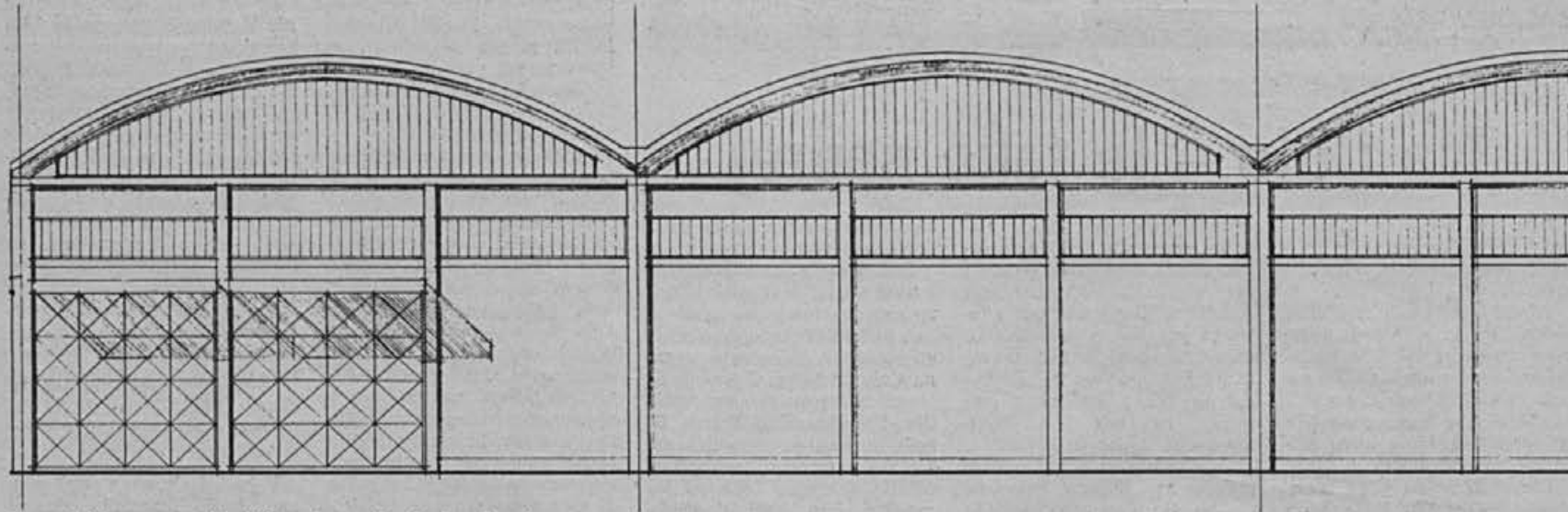
Iz projekta novega skladišča: elementi vzhodne fasade
