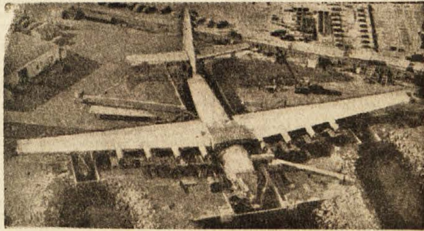
Gradnja gigantskega transportnega osemmotornega letala v Sovjetski zvezi. Letalo meri čez krila 97,5 m in bo nosilo do 350 ljudi naenkrat
