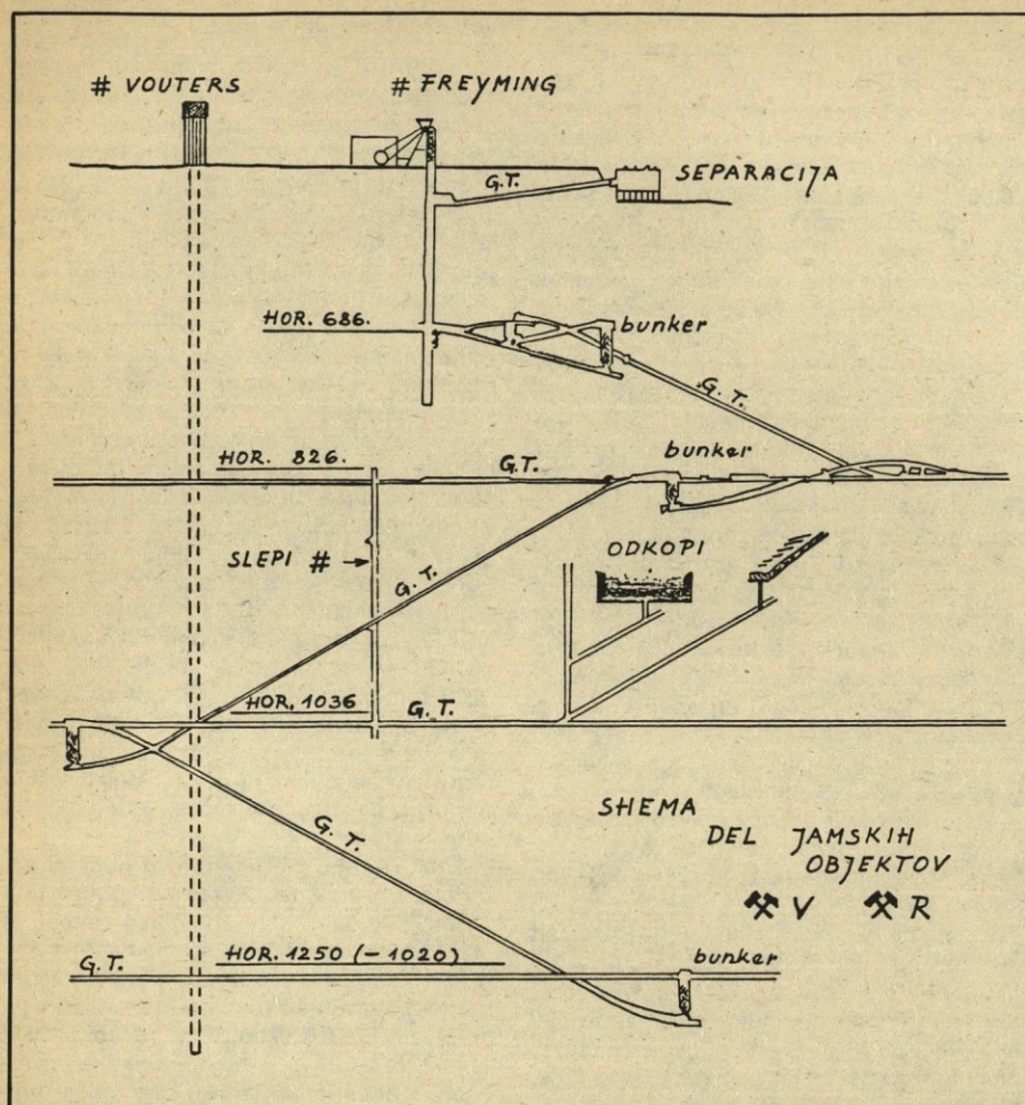
Skica 2 — Shema dela jamskih objektov
