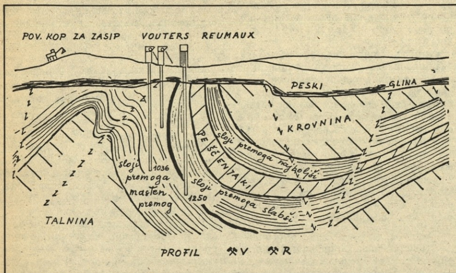
Skica 1 — Površinski kop za zasip
