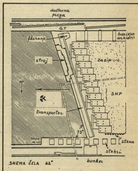
Skica 3 — Shema čela
