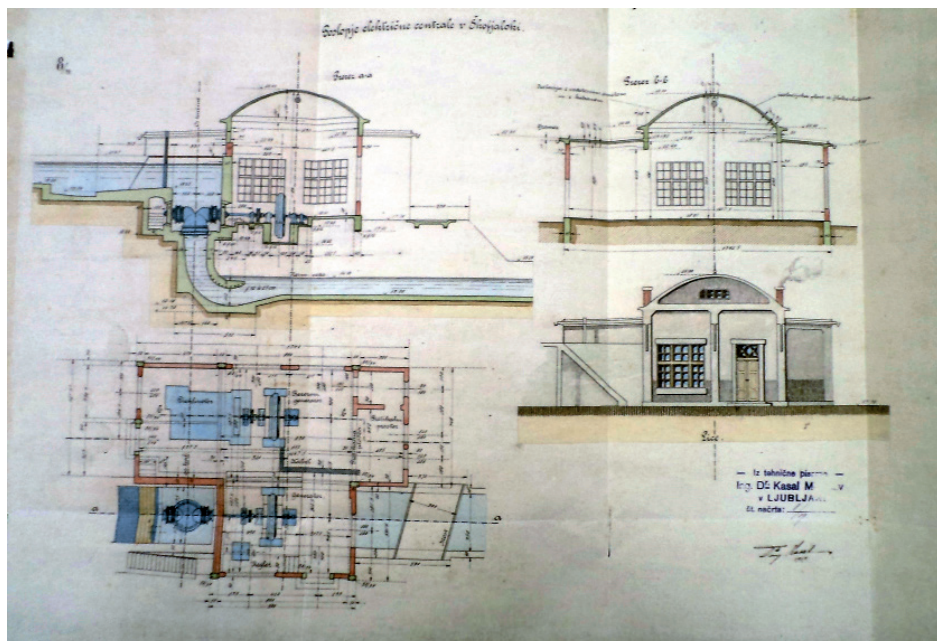
Načrt poslopja in opreme električne centrale v Skalcah na Selški Sori. (hrani: ZAL, Enota v Škofji Loki)
