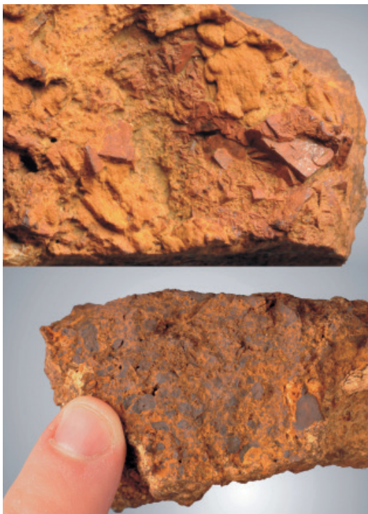
(slika 2) Rudni minerali iz okolice Drage. Ponekod je mogoče zaslediti tudi pseudomorfoze limonita po piritu (zgoraj) in velike kose rude (spodaj). (najdba in foto: Matija Križnar)
