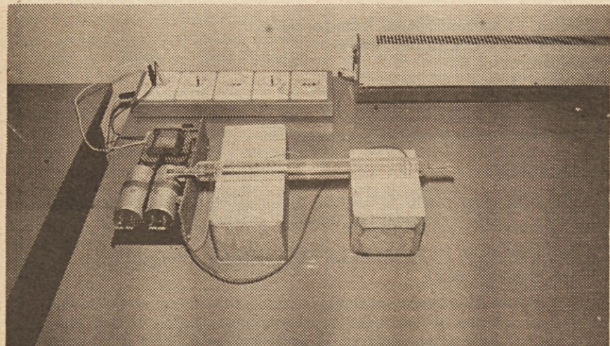
Lastni dosežek - plinska laserska cev.
