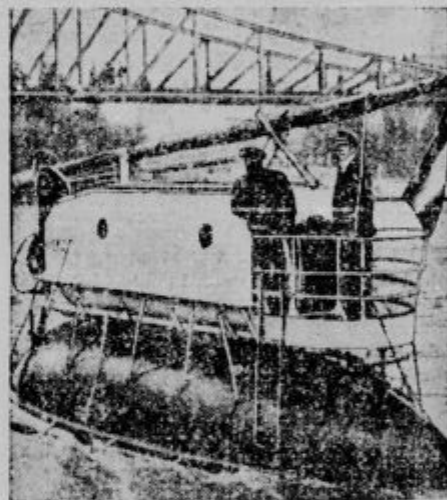
Nepotopljiv rešilni čol, ki ga je zgradil tehnik Albert Sigg v Frankfurtu ob Meni. Čoln more klibovati vsakemu vremenu ter je opremljen z jadrom in motorjem. Njegova brzina znaša do 15 km na uro
