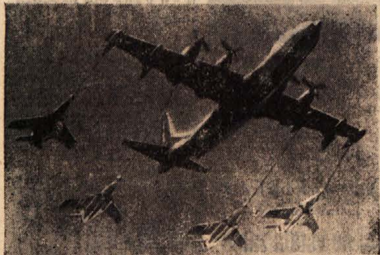
Ameriško letalo Convair R3y-2 »Tradewind« (Pasafni veter) lahko napaja v zraku reaktivne lovce hkrati. Napajanje traja pet minut, letala cisterna na reaktivni pogon pa ima v trupu dovolj goriva za osem lovcev
