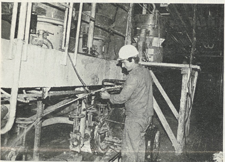
Pranje s pralno napravo WAP — lažje in bolj učinkovito čiščenje strojev in njihove okolice
