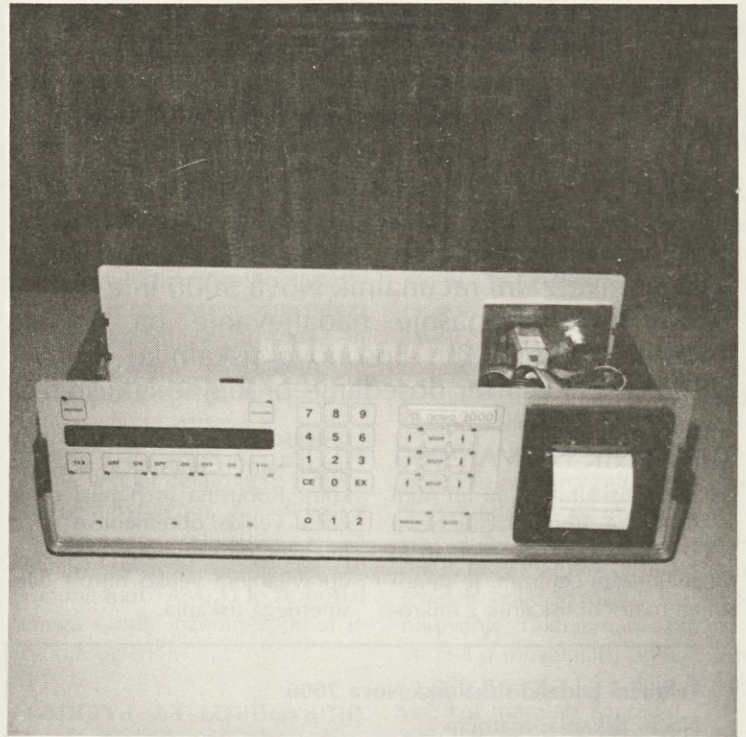
Računalniški sistem Nova 3000
