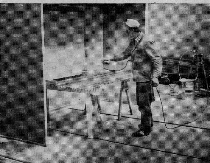
Furnirana krila se lakirajo v traku, letvice za stekla pa se ločeno lakirajo s pištolo kot kaže zgornji posnetek.
