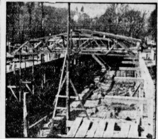
Paviljon ob Celovski cesti gradijo. V ozadju sestavljajo že ogródje ostrešja.
