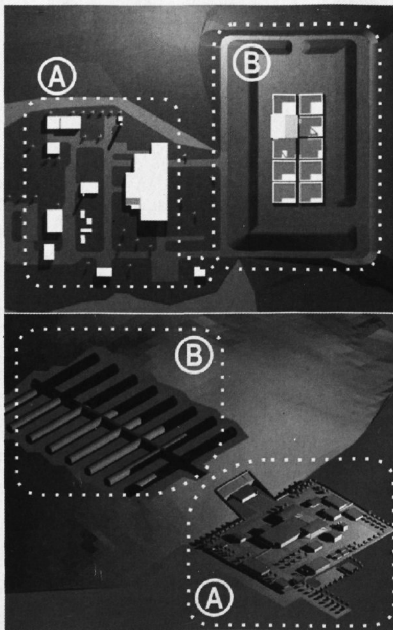
Shematska prikaza površinskega (zgoraj) in podzemnega (spodaj) odlagališča NSRAO iz idejnih projektov Agencije RAO; z A so označena področja pomožnih objektov, z B pa odlagalna območja.
