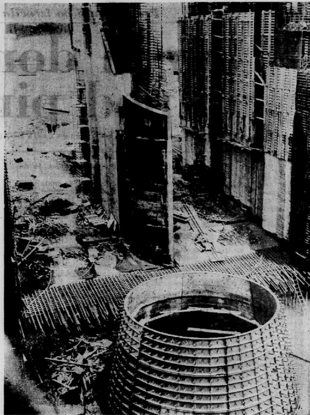
POGLED NA TRETJI AGREGAT
