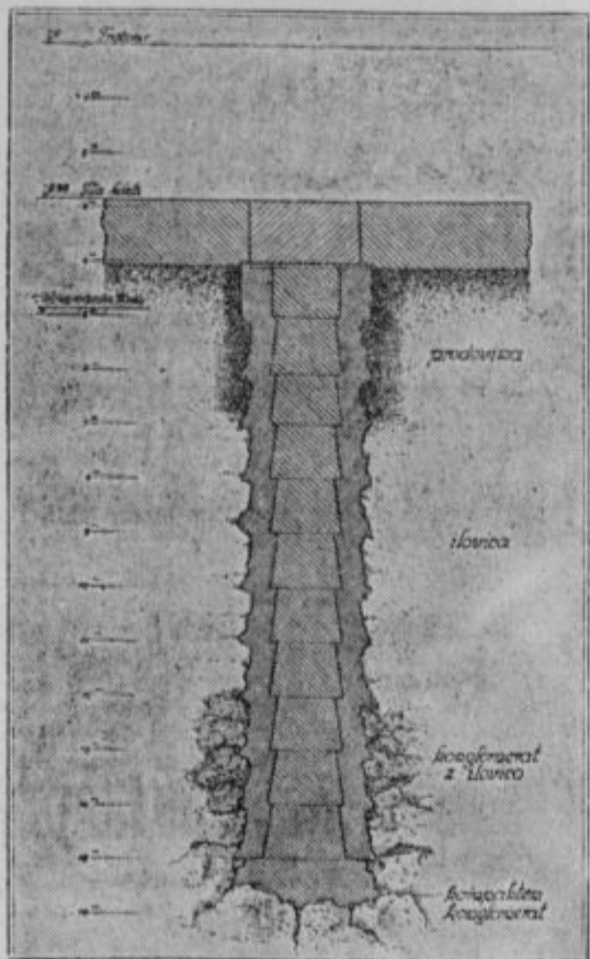
Prerez skozi enega od 16 betonskih stebrov, ki nosijo temelje palače
