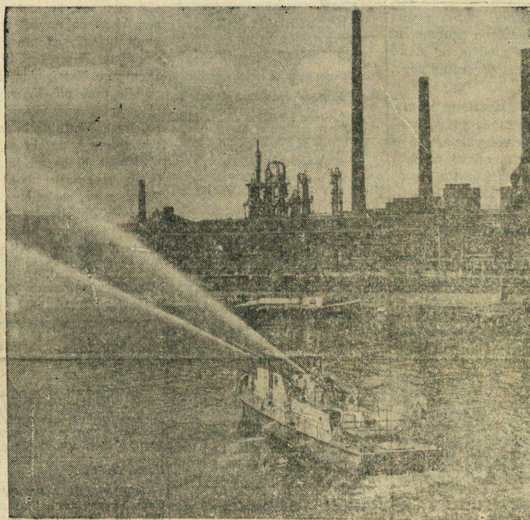
GASILSKA LADJA — Pri Frankfurtu na Renu na Nemškem so nedavno dobili novo gasilsko ladjo, ki je dolga 66 čevljev in ima 52 ton. Njene gasilske cevi in posebni vodni topovi se sposobni pognati vodo daleč na oba bregova. Ladja ne bo gasila samo požare na ladjah in vlačilcih, ampak tudi na zgradbah ob bregovih reke. Na sliki vidimo ladjo pri preskušanju gasilskih naprav.
