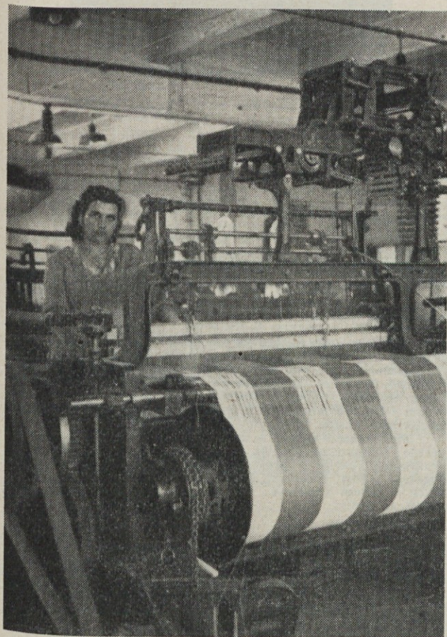
Tisoči artikel na stroju
