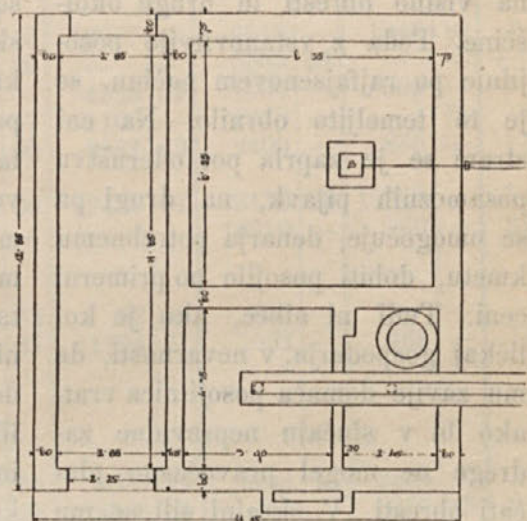
Slika D. Temeljni tloris.
