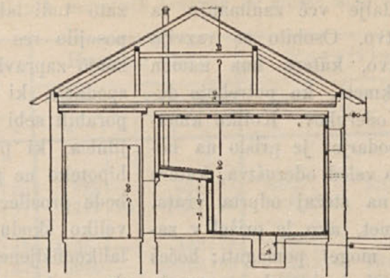
Slika B. Prerez a—b.
