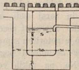
Slika E Detajl greznične omare \frac{1}{50} nar. velikosti.
