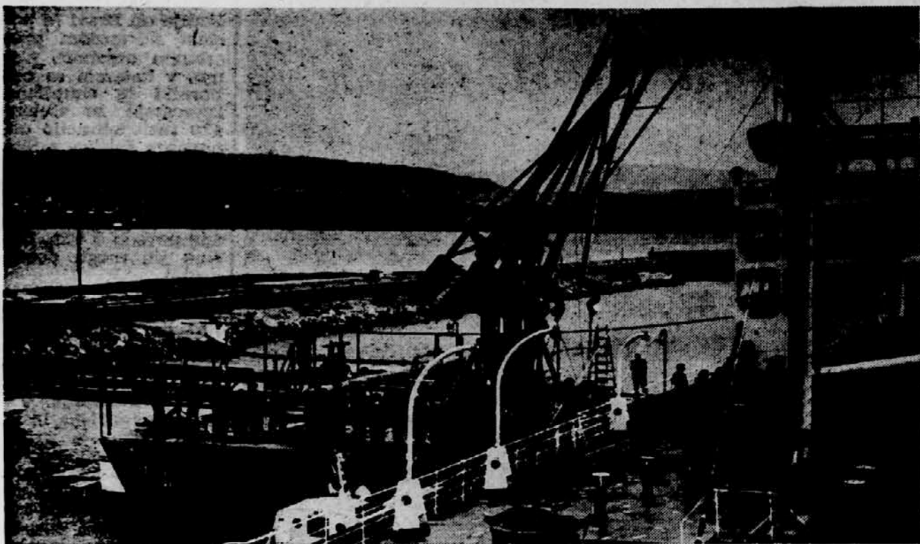
PRISTANIŠČE ZA TEKOČE TOVORE — Pomol pristanišča za tekoče tovore v koprski luči prepletajo številne cevi. Ko ladja pristane ob pomolu, pritrdijo s pomola črpalne cevi na ladijske cevrode. Črpalke poženejo po ceveh na uro tudi do 1000 ton nafte. V ozadju je videti nasip s skoraj dva in pol kilometra dolgim cevovodom do cistern na pobočju Sermina.
