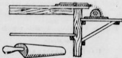
Sl. 12. Priprave za izdelavo slemenjakov.
