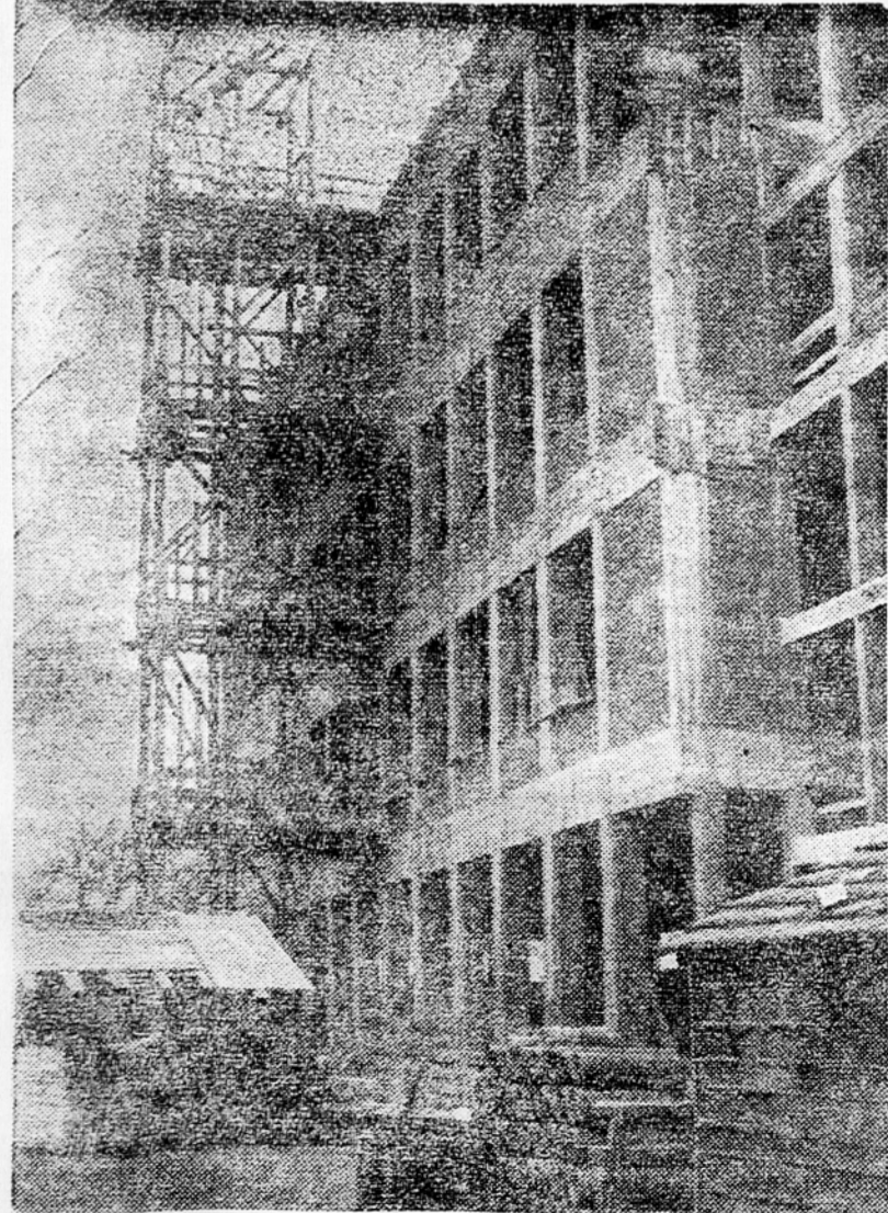
Na gradbišču bodoče poštne palače v bližini glavnega kolodvora v Ljubljani je delo zadnje tedne oživel. Gradnja je od lanskega leta počivala, ker je češkoslovaška tovarna v Šlesku odpovedala pogodbo o dobavi nove telefonske centrale. Sedaj, ko je dobava telefonske centrale iz druge države zagotovljena je treba delo pospešiti, da bo do julija prihodnjega leta vse pripravljeno za montažo nove telefonske centrale.
