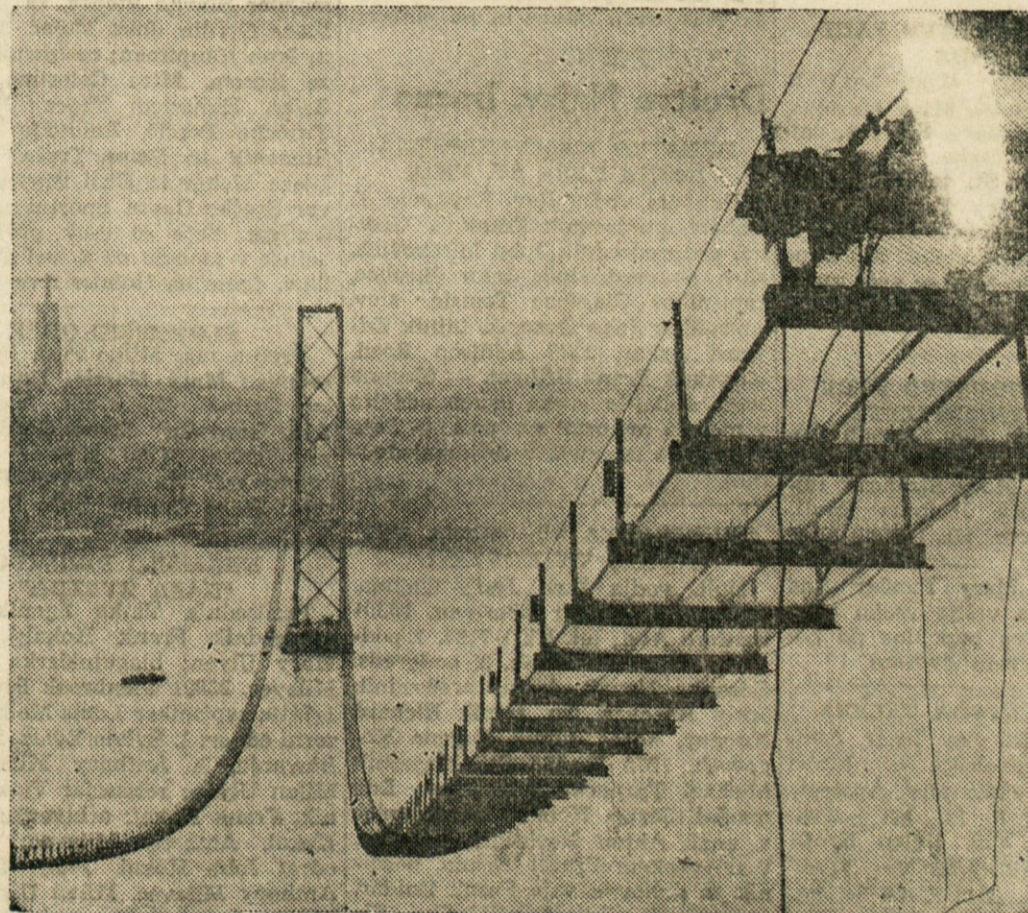
VIŠEČI MOST GRADE PREKO TAGU — Slika kaže gradnjo višičnega mostu čez reko Tagu v glavnem mestu Portugalske Lizboni. Most bo najdaljši svoje vrste v Evropi, saj bo meril 3.323 čevljev.
