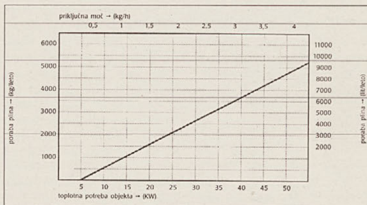
Določitev okvirne letne porabe plina z ozirom na energetske potrebe objekta
