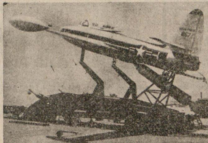
Pred vzletom: ameriški F-84 »Thunderjet« (ki jih ima tudi jugoslovansko vojno letalstvo) se dviga na »roke« priklopnika v položaj za vzlet. Od zadnjega dela trupa mu visi velika raketa, ki mu omogoča dvig »z najmanjšega letališča na svetu«
