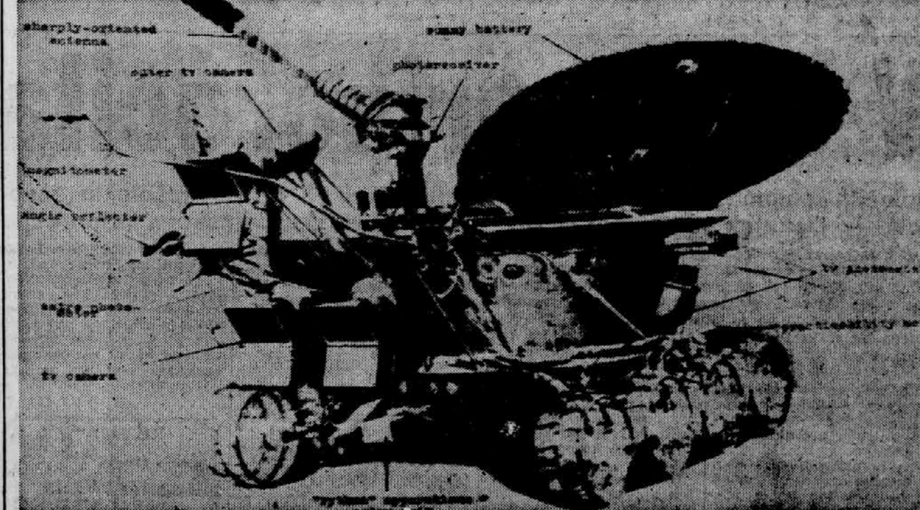
LUNARNO VOZILO — Kot smo že poročali je sovjetska avtomatska postaja Luna 21 mehko pristala na Luni. Iz nje je sestopilo avtomatično vozilo Lunohod 2, ki je takoj opravilo nekaj poskusnih voženj. Kakšno je to vozilo, vidimo na sliki. Telefoto: "ASS"
