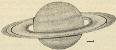
Saturn s kolobarjem (—| Zemlja v primeri s Saturnom)
