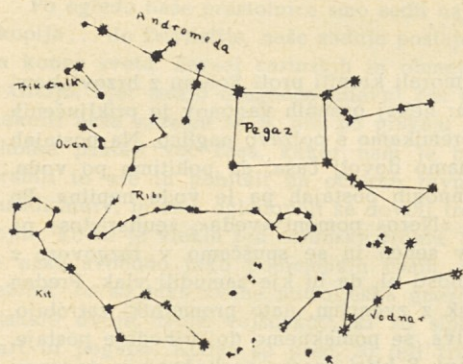
Saturn je 1. 1939. v Ribah (Ozvezdje v mesecu januarju in februarju na jugozapadnem nebu)
