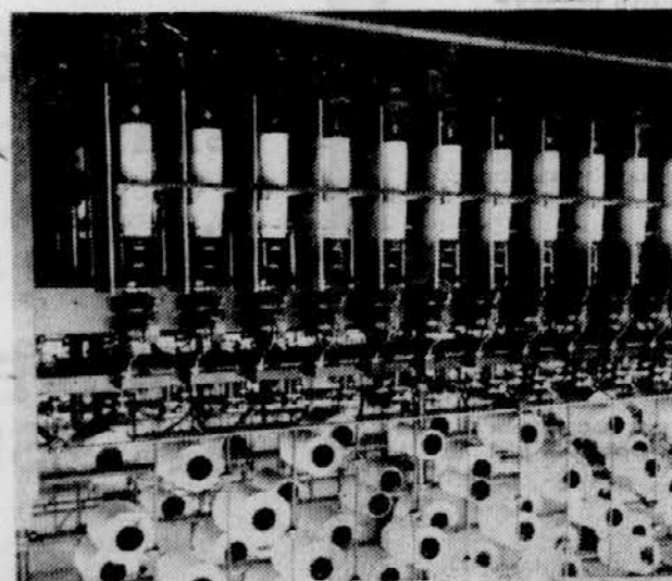
Detajl iz dvojilnice
