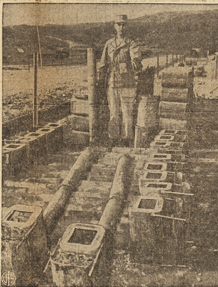
BORBA Z "MRZLO" VOJNO NA KOREJI — Častnik Angelo Fabrice iz Geneva, N. Y., ki je izdelal načrt za 1952 vzorec peč za ogrevanje zaklonišč na korejskem bojišču, kaže na zalogo teh izdelkov. Peči so izdelane iz nerabnih kovinastih zabojev za topovsko municijo in se jih lahko kuri z drvmi, premogom, oljem ali bencinom.
