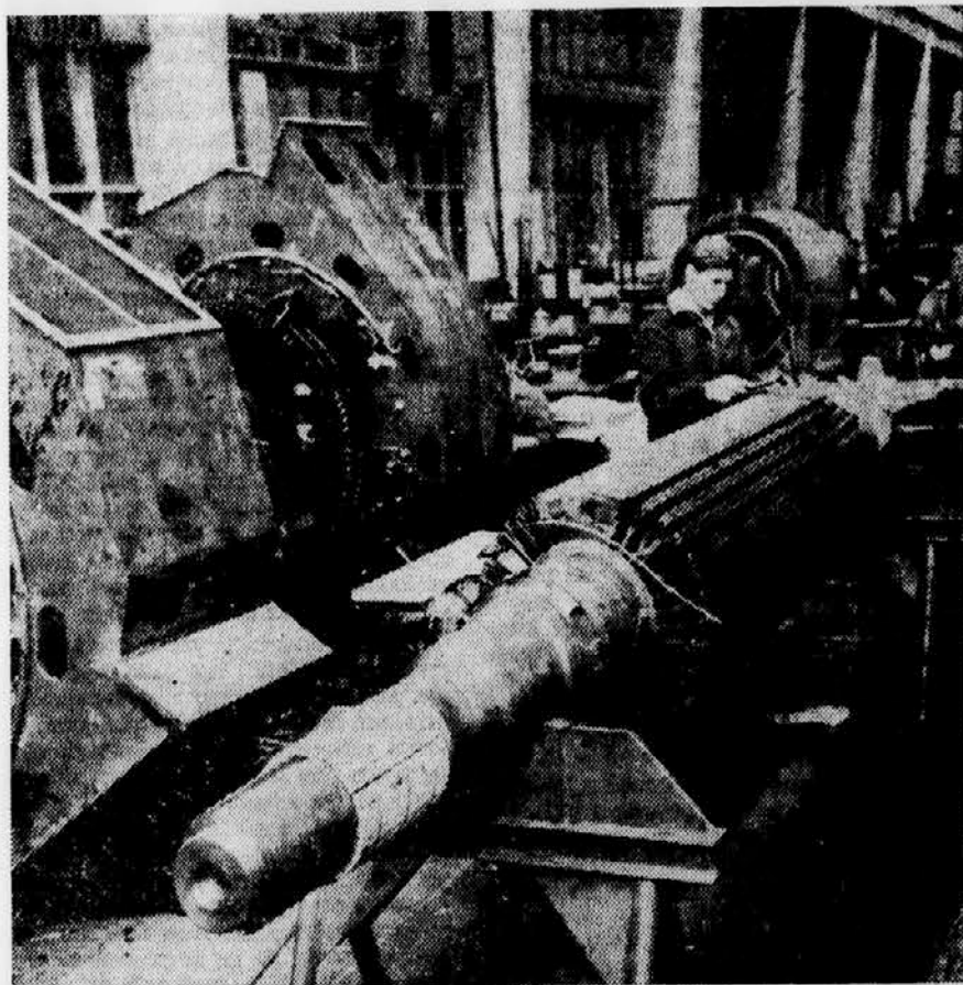
Proizvodnja generatorjev v tovarni »Rade Končar«
