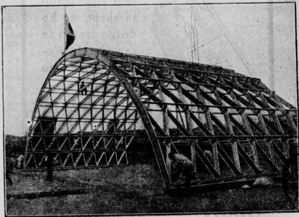
Streha brez opornih stebrov. Na tehničnem velesojmu v Leipzigu je razstavil prof. Junker 60 m široko in 20 m visoko strešno ogrodje, ki ne potrebuje opornih stebrov. Konstrukcija je primerna predvsem za zrakoplovne lope in kmetijska gospodarska poslopja.
