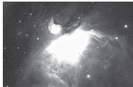
Orionova meglica M42, znana kot porodnišnica zvezd
