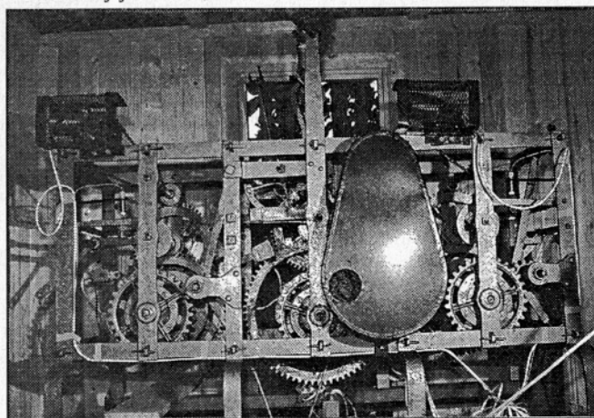
Pogonski mehanizem stolpne ure v delavnici Uroša Aubrehta (foto: Sašo Bernardi)
