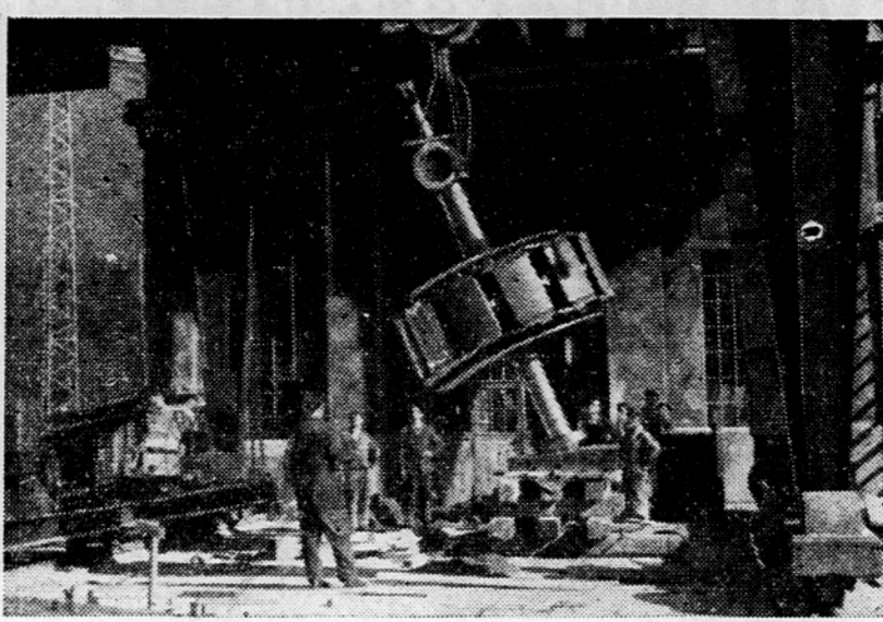
Stroje v hidrocentrali Moste je postavila ekipa monterjev mariborske »Hidromontaže«. Na sliki vidimo, kako s pomočjo portalnega žerjava spuščajo v strojnico rotor velikega generatorja.
